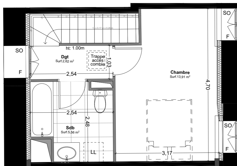
Duplex haut
