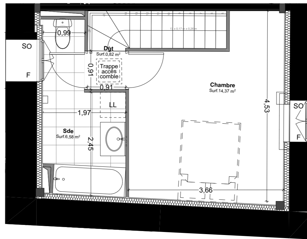
Duplex haut
