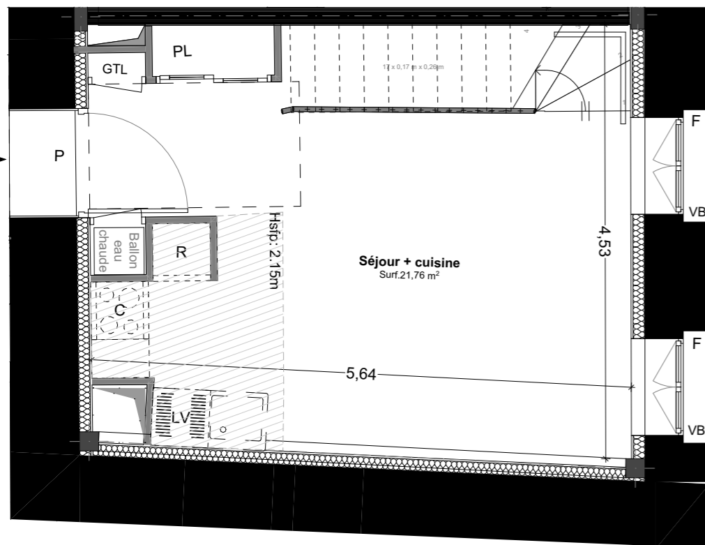
Duplex bas (accès R+1)
